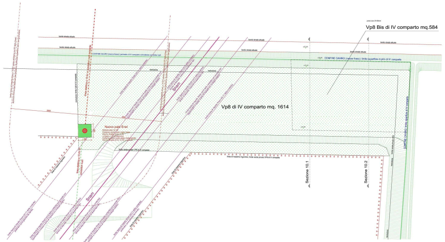
Stato modificato scala 1:200
