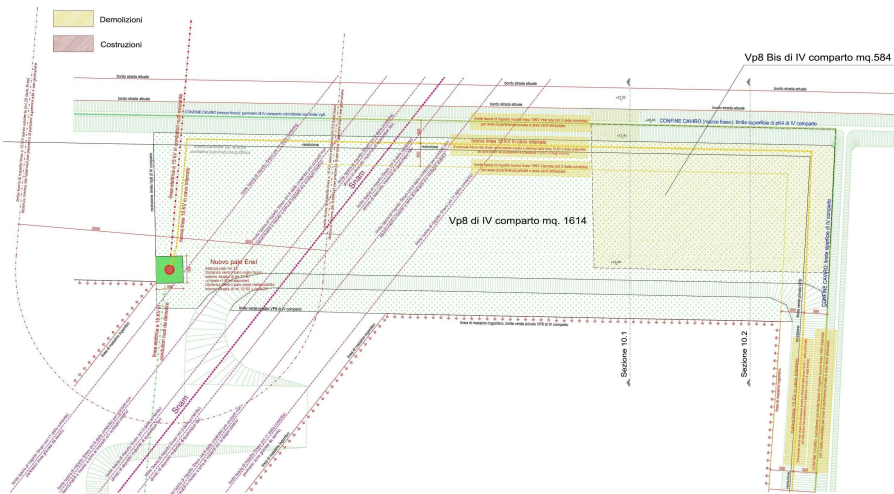
Stato comparato scala 1:200
