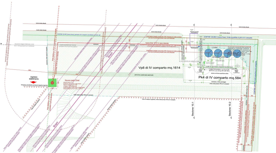
Stato attuale scala 1:200
